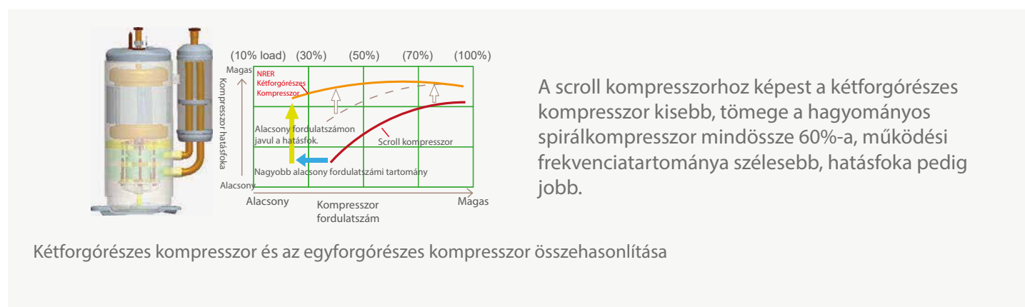
Kétforgórészes kompresszor és az egyforgórészes kompresszor összehasonlítása
